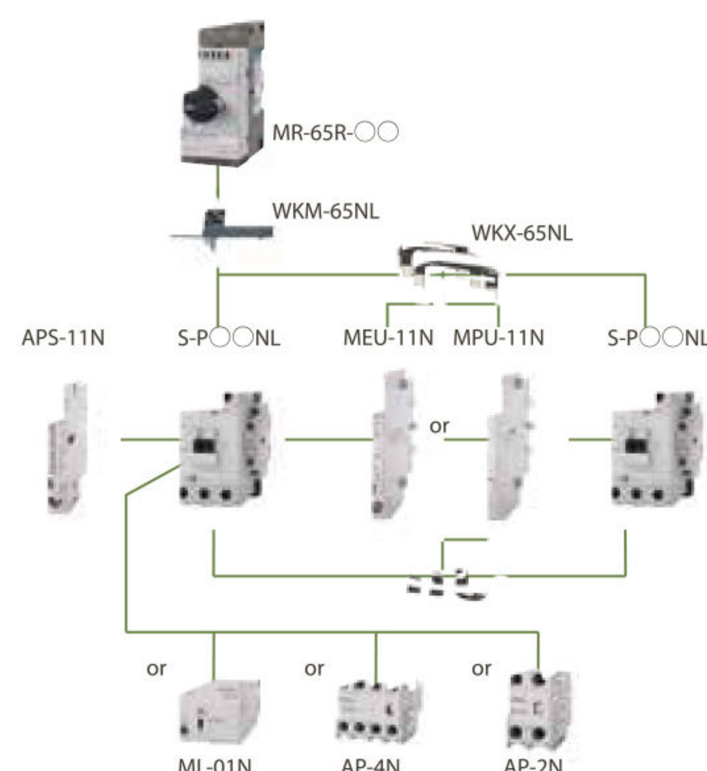
MMS+MS-N應用例圖 MR-65R系列
